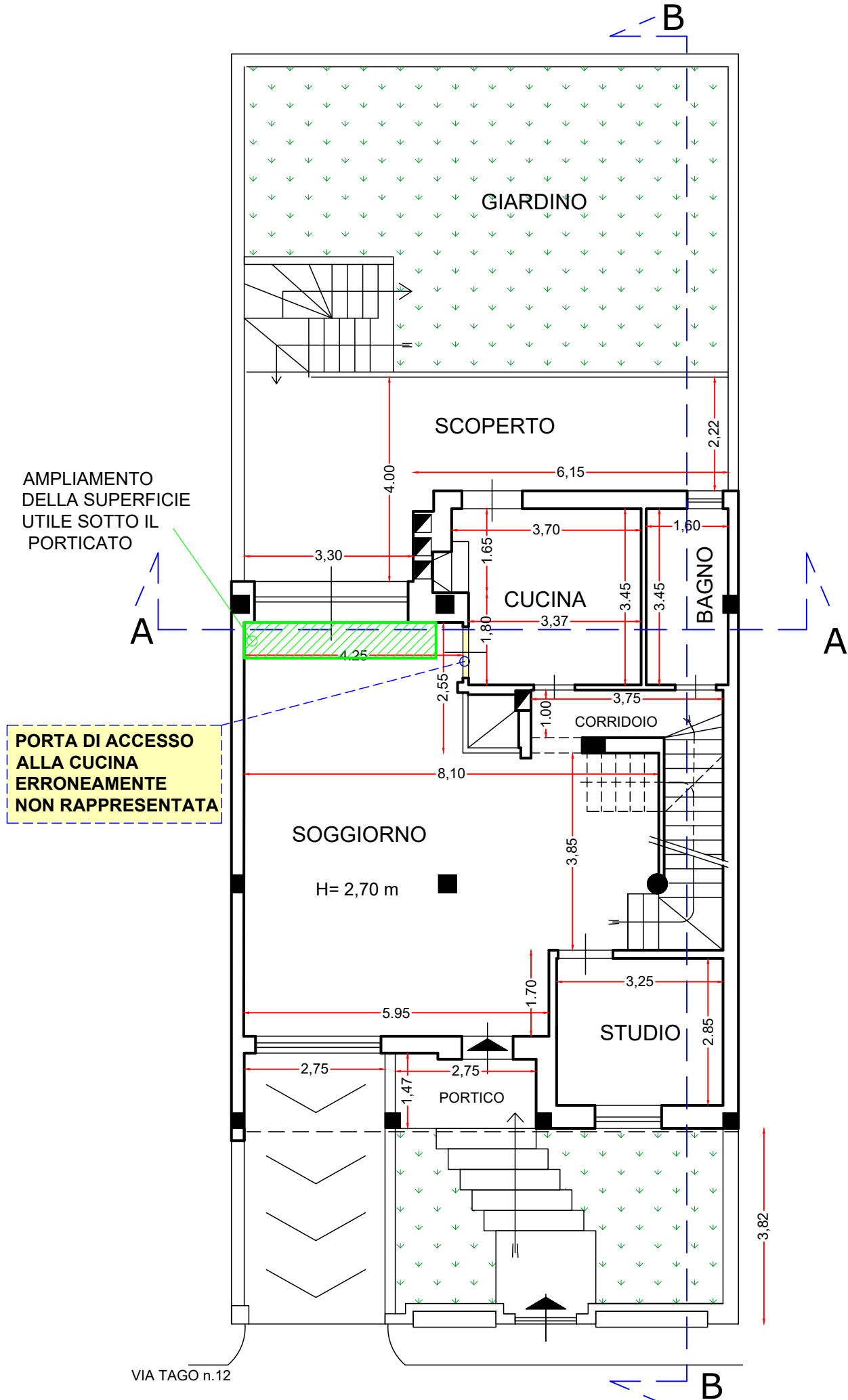
PIANTA PIANO PIANO TERRA - 1:100 IN VARIANTE NON ESSENZIALE
