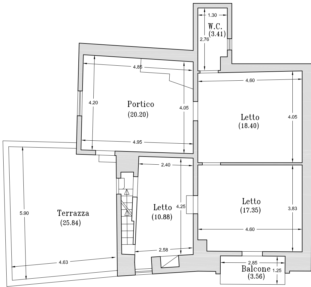
PIANO PRIMO
